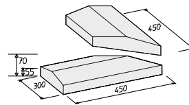
Mauerabdeckung Ecke Dachform, 2-teilig
