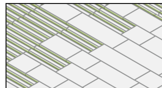
Padio® 20, Reihenverband mit Hydropor Padio Rasenplatte oder Rasenfugenstein
