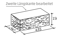
Endstein
