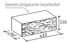
Brüstungsstein
