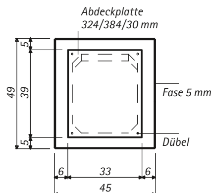
Vorderansicht
