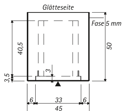
Draufsicht
